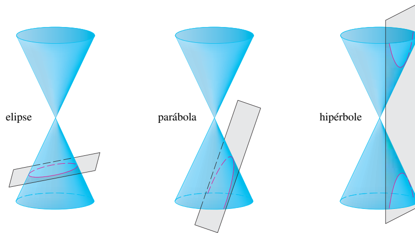
FIGURA 1 Cônicas
