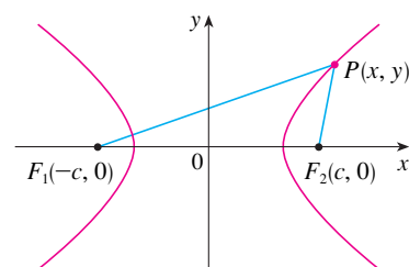
FIGURA 11 P está na hipérbole quando |PF_1| - |PF_2| = \pm 2a .
