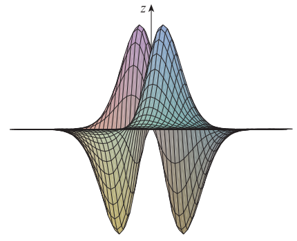
(b) Duas vistas de f(x, y) = -xye^{-x^2-y^2}
