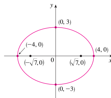
FIGURA 10 9x^2 + 16y^2 = 144
